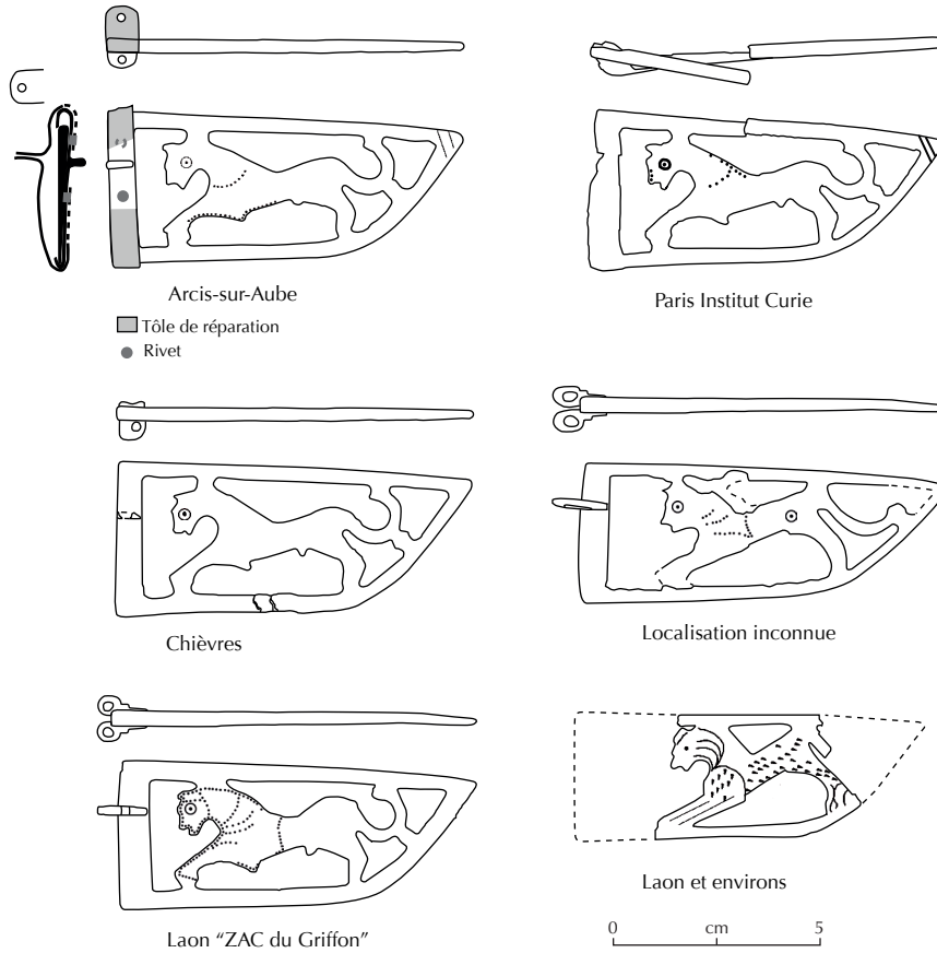
Fig. 4. Le couteau à fourreau à décor zoomorphe ajouré d'Arcis-sur-Aube et les parallèles connus (cl. M. Brunet, dessins B. Fort et M. Brunet).
