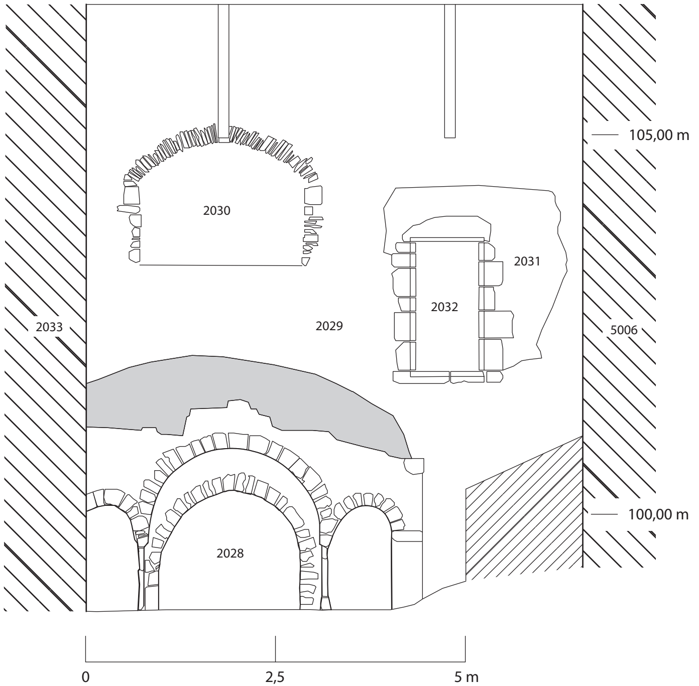
CHATEAU DE FOUGERES - LOGIS Salle 2 élévation sud
