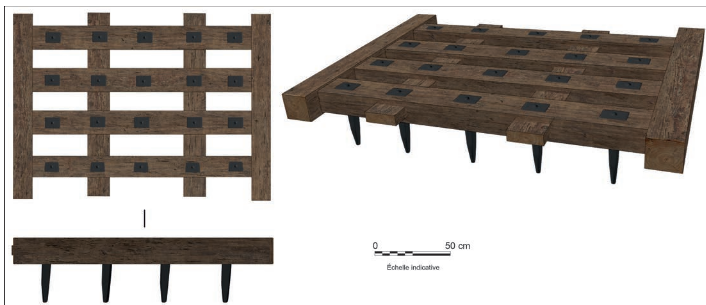
Fig. 10 – Essai de restitution de la herse de Contrexéville (modélisation : É. Chabrol).
