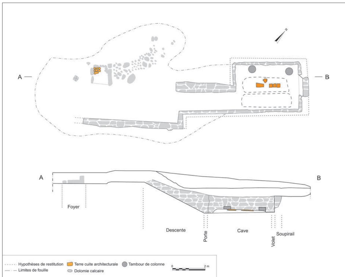
Fig. 2 – Plan et coupe de la cave du site de la Côte, d'après les relevés du Cercle d'études locales de Contrexéville (DAO : G. Huitorel, UMR 7041).
