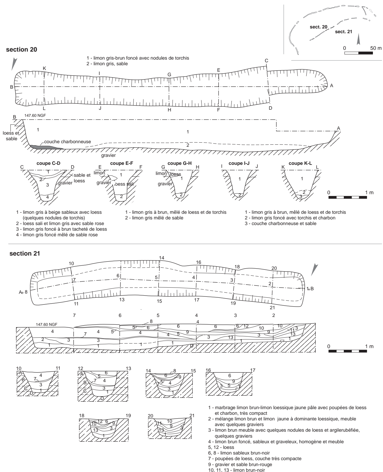
Fig. 109: Entzheim « Les Terres de la Chapelle » : coupes transversales et longitudinales des sections 20 et 21 de l'enceinte. © P. Lefranc, P. Girard, Inrap.
