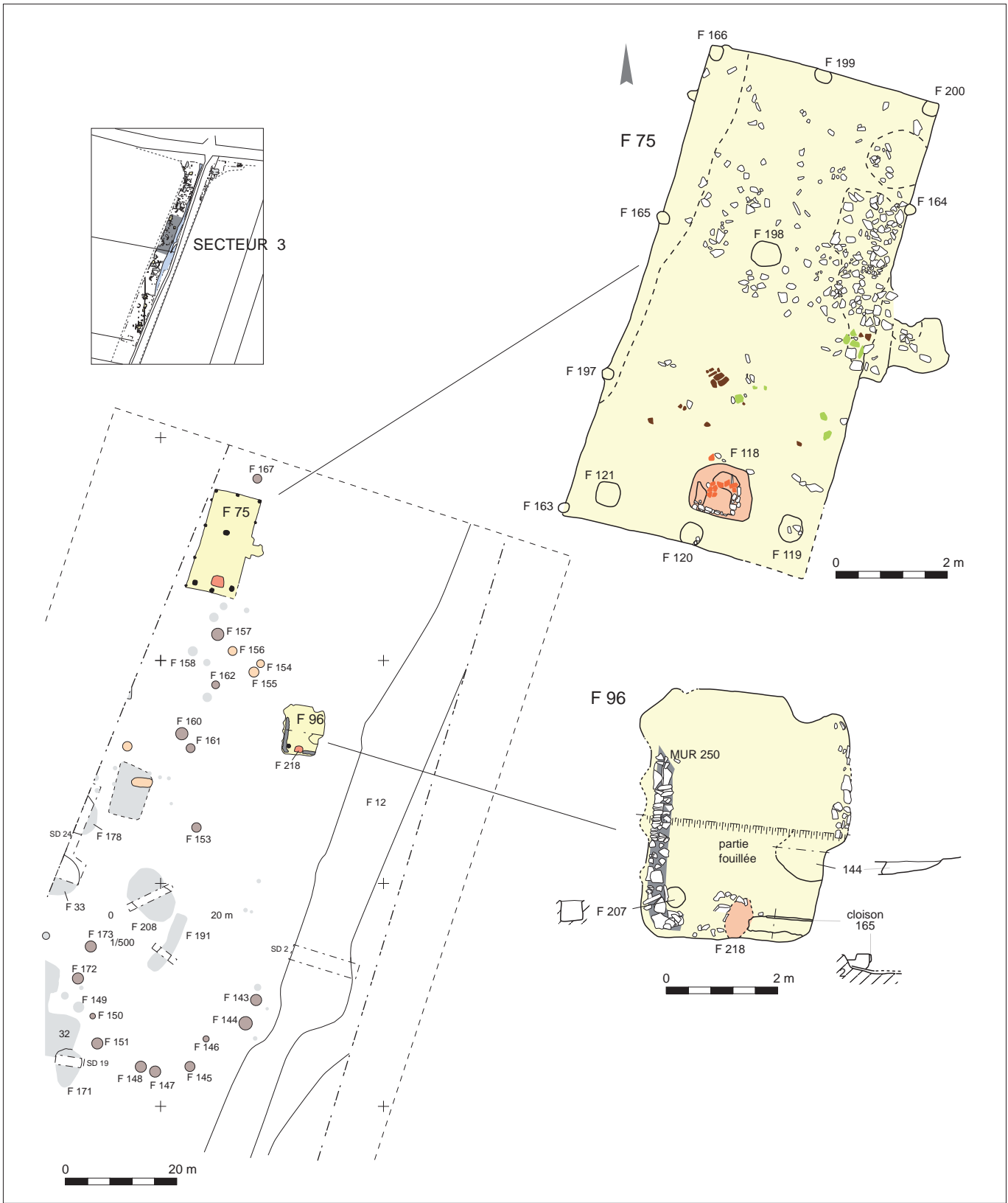
Fig. 8. Plans des bâtiments F75 et F96. © G. Alfonso, DAO É. Rouger.
