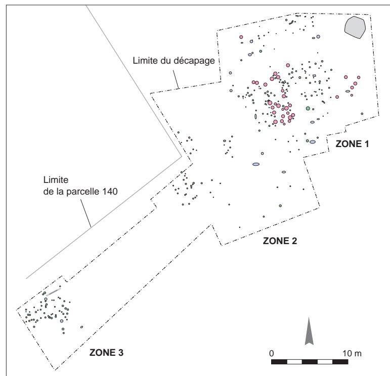
Fig. 1. Plan d'ensemble des vestiges. © D. Parent.
