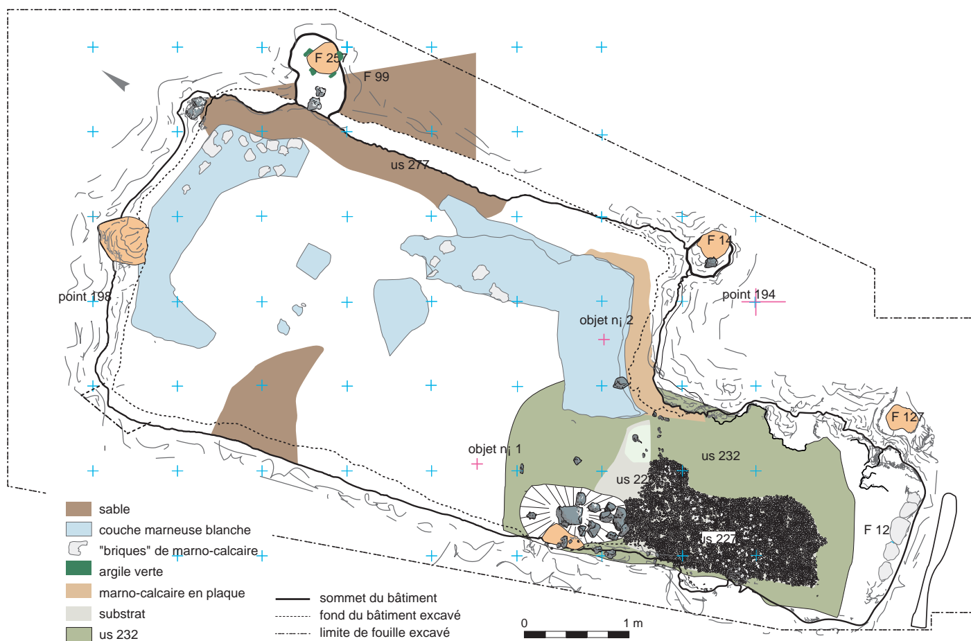
Fig. 3. Plan et coupe du bâtiment F95-état 2. © S. Gaime.
