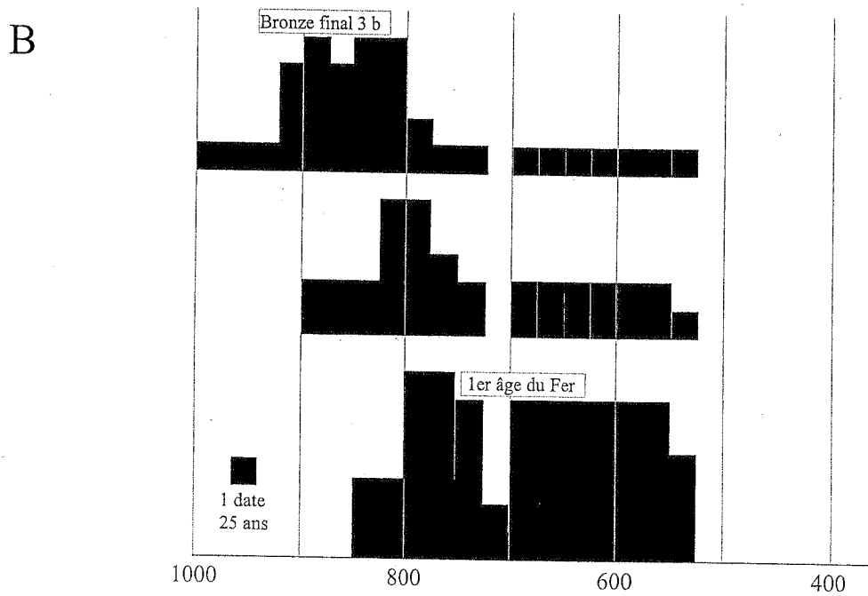
Fig. 8. L'apport des datations 14 C : situation chronologique du faciès Saint-Sorlin/Sermérieu/Les Perches entre le Bronze final IIIb et le Premier âge du Fer type Pré de la Cour / phase 1. A : dates calibrées à 1 écart-type. B : diagramme cumulatif non pondéré par tranches de 25 ans. Dessin F. Thiériot, Inrap.
