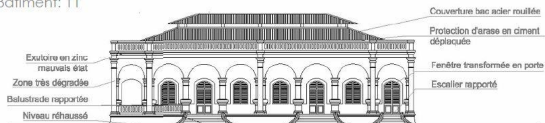
Élévation est
