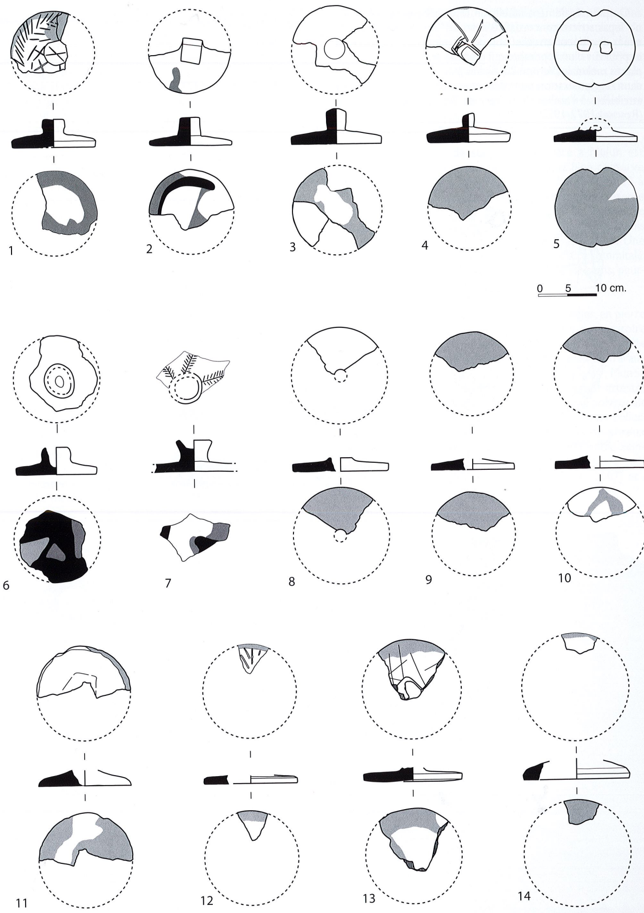
Fig. 3 – Les couvercles plats (profil, vue des faces supérieure et inférieure). En trame, les traces de chauffe plus ou moins importantes (Dessins : M. Queffurus : n° 2, 6 et 7 ; V. Pissot : n° 1, 3 à 5, 8 à 14). Provenance : Melun, excepté n° 3 (Moissy-Cramayel), n° 4, 10, 11 et 14 (Avon), n° 8 (Lieuxaint).
