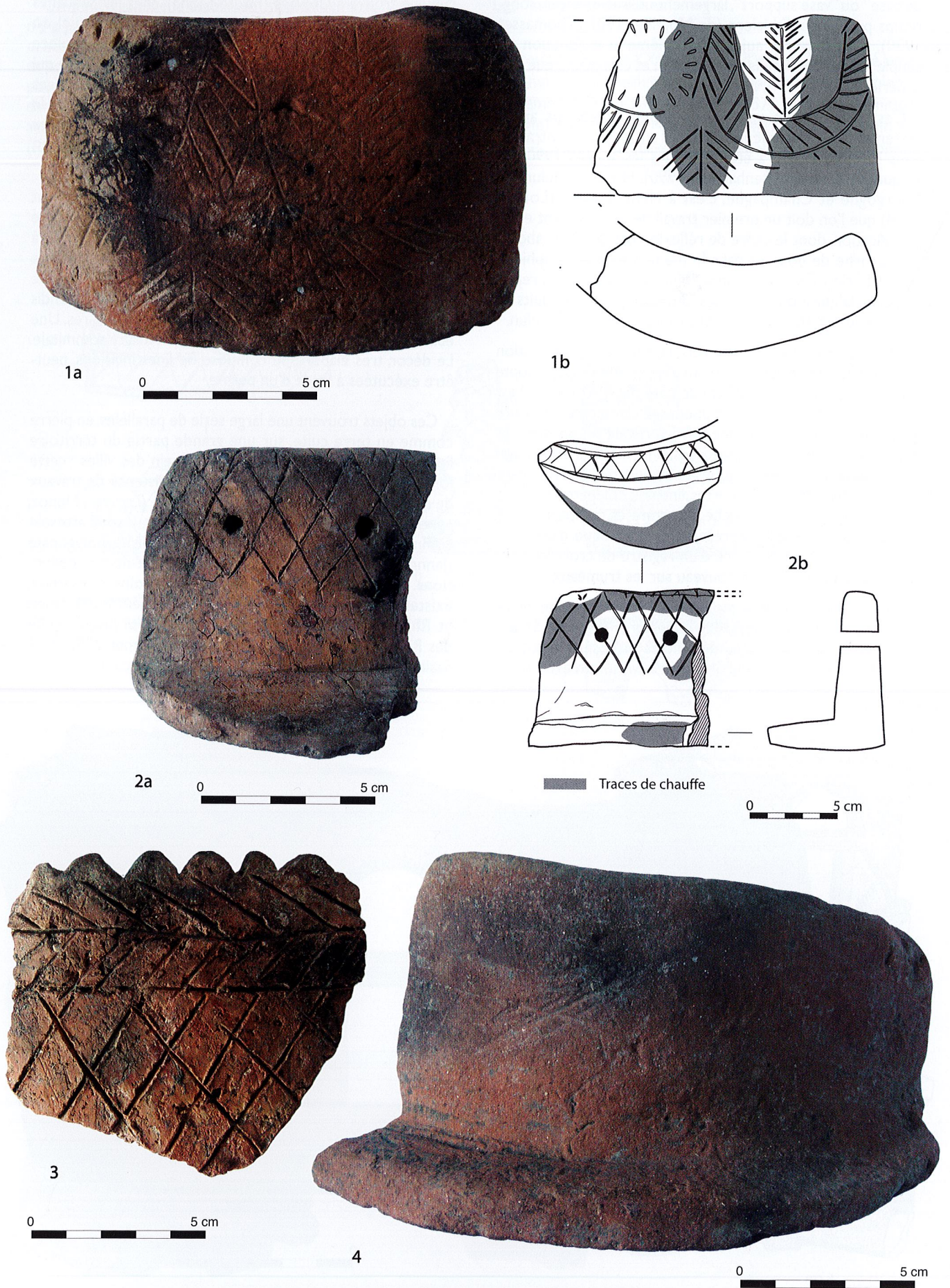
Fig. 6 – Quatre objets courbes de Melun (n° 1 à 3) et de Lieusaint (n° 4) [Clichés :V. Pissot ; dessins : O. Blin (n° 1b) et V. Pissot (n° 2b)].
