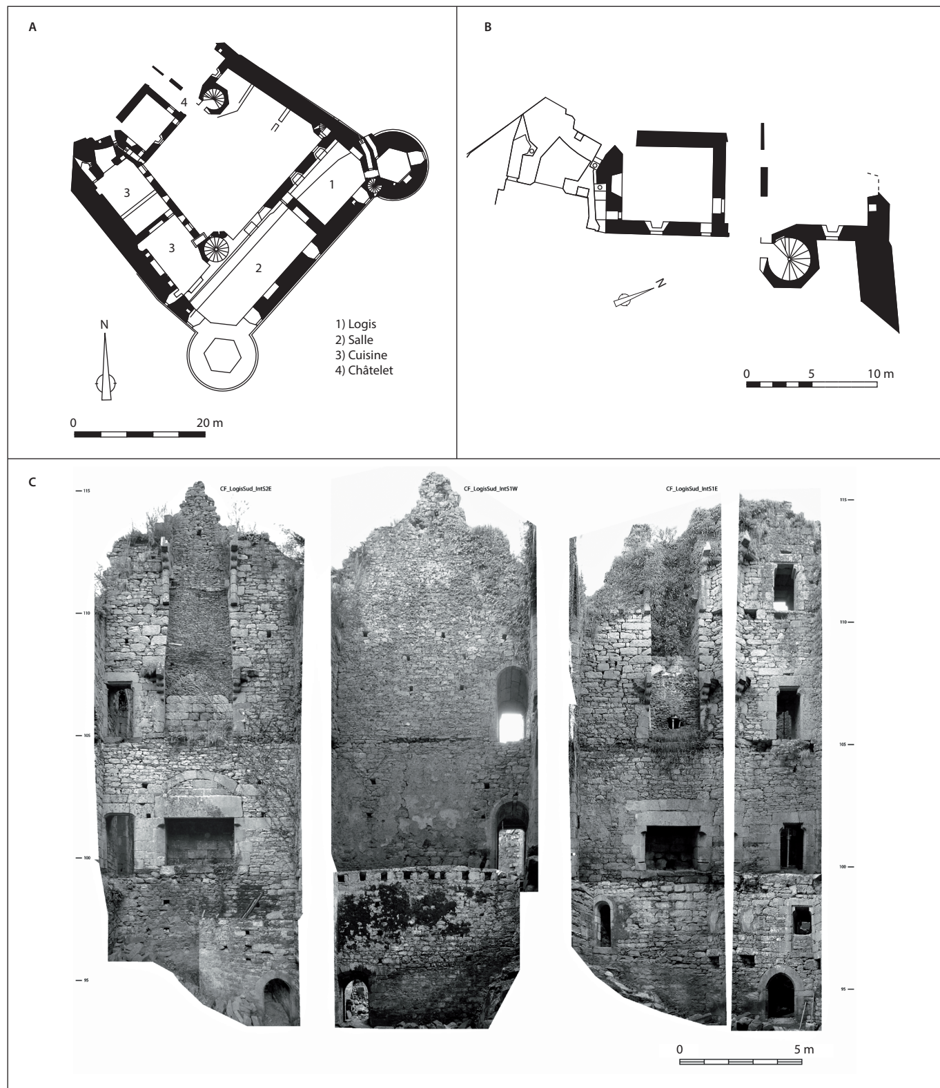
Fig. 5 A) plan du château de Coatfrec (doc. F. Boumier, Inrap); B) détail du plan des vestiges du châtelet (doc. F. Boumier, Inrap); C) orthophotographies des élévations du mur de refend et du pignon oriental du grand logis (doc. et clichés F. Boumier, Inrap).
