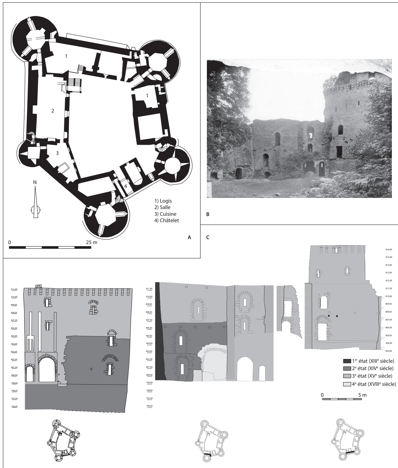
Fig. 4 A) plan du château de la Hunaudaye (doc. E. Esnault) ; B) vue des vestiges de l'entrée au début du XX e siècle (© ministère de la Culture, médiathèque de l'Architecture et du Patrimoine, dist. RMN-GP) ; C) levé des élévations subsistant et proposition de chronologie (doc. E. Esnault).
