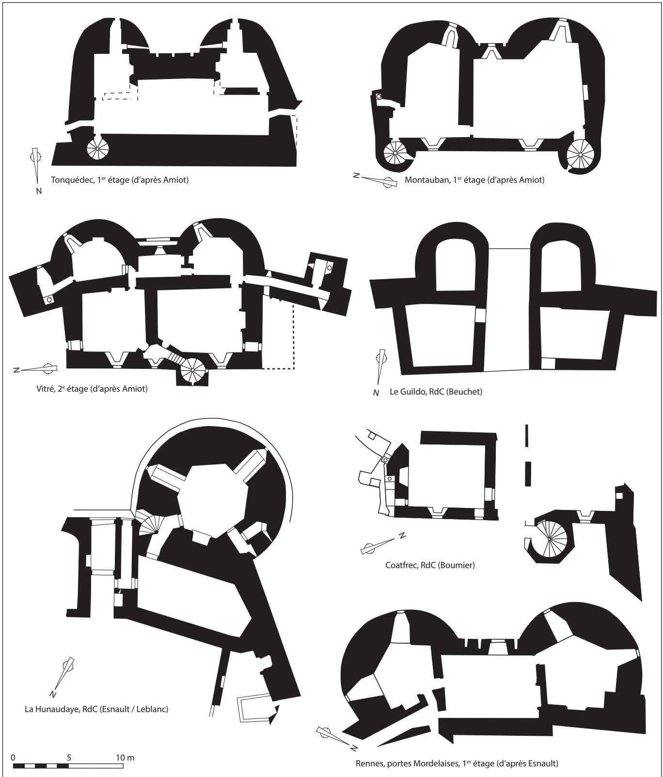
Fig. 6 Plans des principaux châtelets mentionnés dans le texte. Doc. L. Beuchet.
