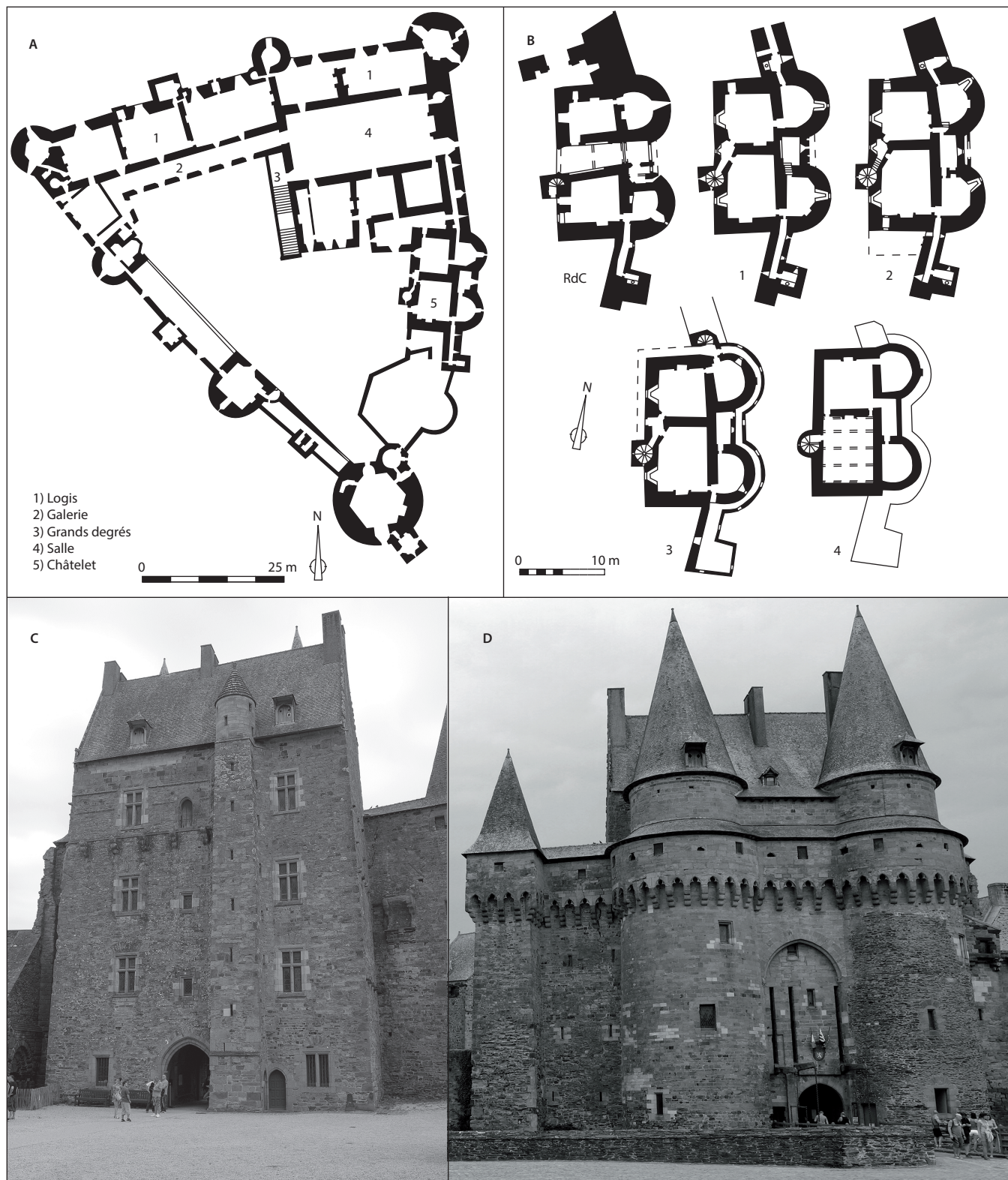
Fig. 2 A) plan du château de Vitré, d'après Dehuz (© musée de Vitré); B) plan des cinq niveaux du châtelet du château de Vitré, d'après C. Amiot (AMIOT 1998); C) élévation occidentale du châtelet, on note les vestiges de coursière au quatrième niveau, et les supports d'une extension à pans de bois au second niveau, au sud, ainsi que sa cheminée (cliché L. Beuchet); D) élévation orientale du châtelet, on note la tourelle carrée des latrines, au sud (cliché L. Beuchet). Infographie L. Beuchet.
