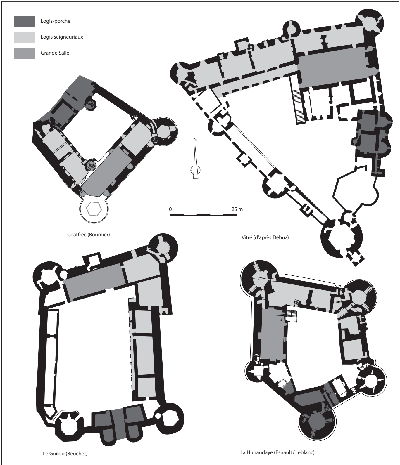
Fig. 7 Plan comparé des principaux châteaux étudiés, présentant la répartition des fonctions résidentielles et de représentation. Doc. L. Beuchet.
