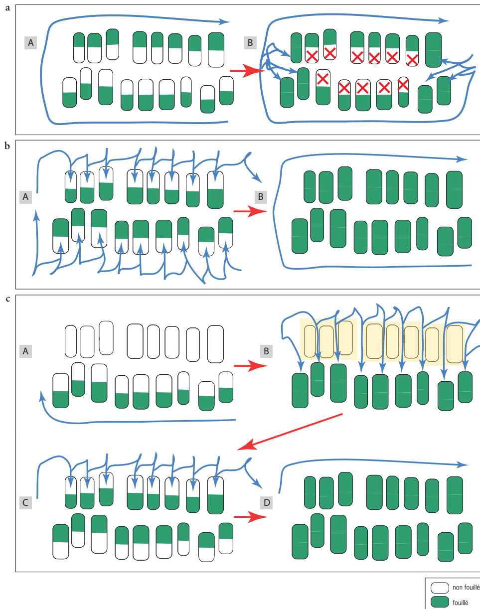
Fig. 2. (a) Éviter de circuler sur une partie des structures conduit à traiter manuellement de nombreuses parties devenues inaccessibles aux engins (croix rouges). (b) Commencer par les parties les moins accessibles permet de réduire les contraintes et d'optimiser l'utilisation d'une mini-pelle. (c) Renoncer à fouiller l'ensemble des fosses en même temps et mettre en place des protections (feutre géotextile, en B) permet d'optimiser la fouille mécanisée tout en intégrant ici une condition particulière : aborder systématiquement la partie basse de chaque structure.
