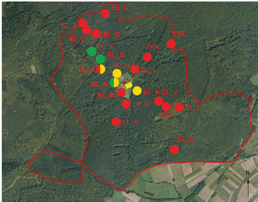
FIGURE 5 SPATIALISATION DES RÉSULTATS DE L'ANALYSE DES SOLS PAR SPECTROSCOPIE PROCHE INFRAROUGE
