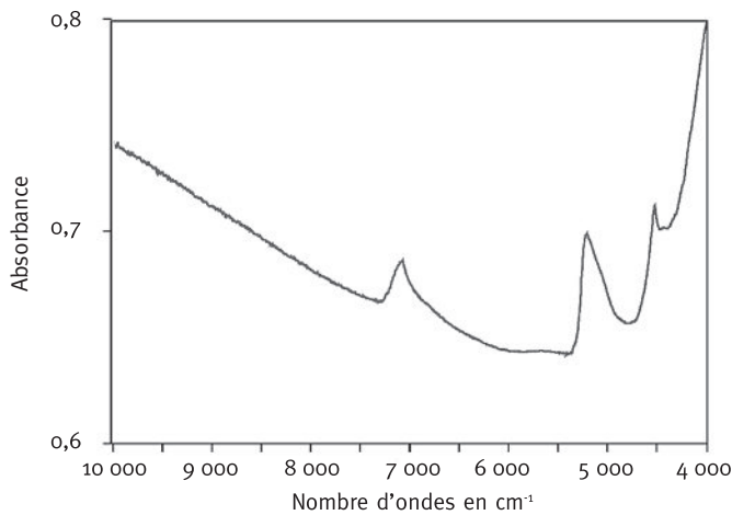
FIGURE 2 EXEMPLE D'UN SPECTRE PROCHE INFRAROUGE MESURÉ SUR UN ÉCHANTILLON DE SOL ET TRANSFORMÉ EN ABSORBANCE (A)
