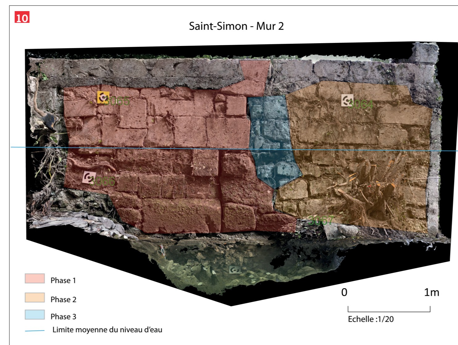
10. Traitement photogramétrique sur le site de Saint-Simon (16) Les différentes phases du mur. P. Sauer, O. Dapens, Inrap.
