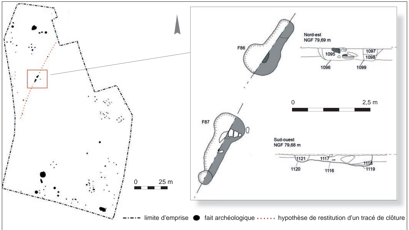
▲ Fig. 68. Plan de répartition des vestiges de LT A1 des Chauffeaux à Sainte-Maure-de-Touraine, Indre-et-Loire, phase 1 (d'après Di Napoli, Lusson, 2011, fig. 5). Exemple d'un établissement rural dont le probable enclos n'est matérialisé que par l'ancrage au sol d'un système d'accès renforcé (structures F86 et F87).
