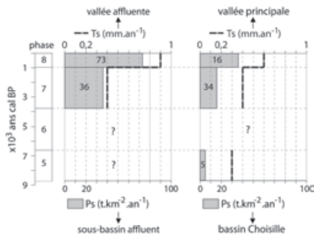
Figure 8: Taux de sédimentation (Ts en \text{mm}\cdot\text{an}^{-1} ) et production sédimentaire solide minimale (Ps en \text{t}\cdot\text{km}^2\cdot\text{an}^{-1} ) estimés d'après les stocks sédimentaires en fond de vallée.
