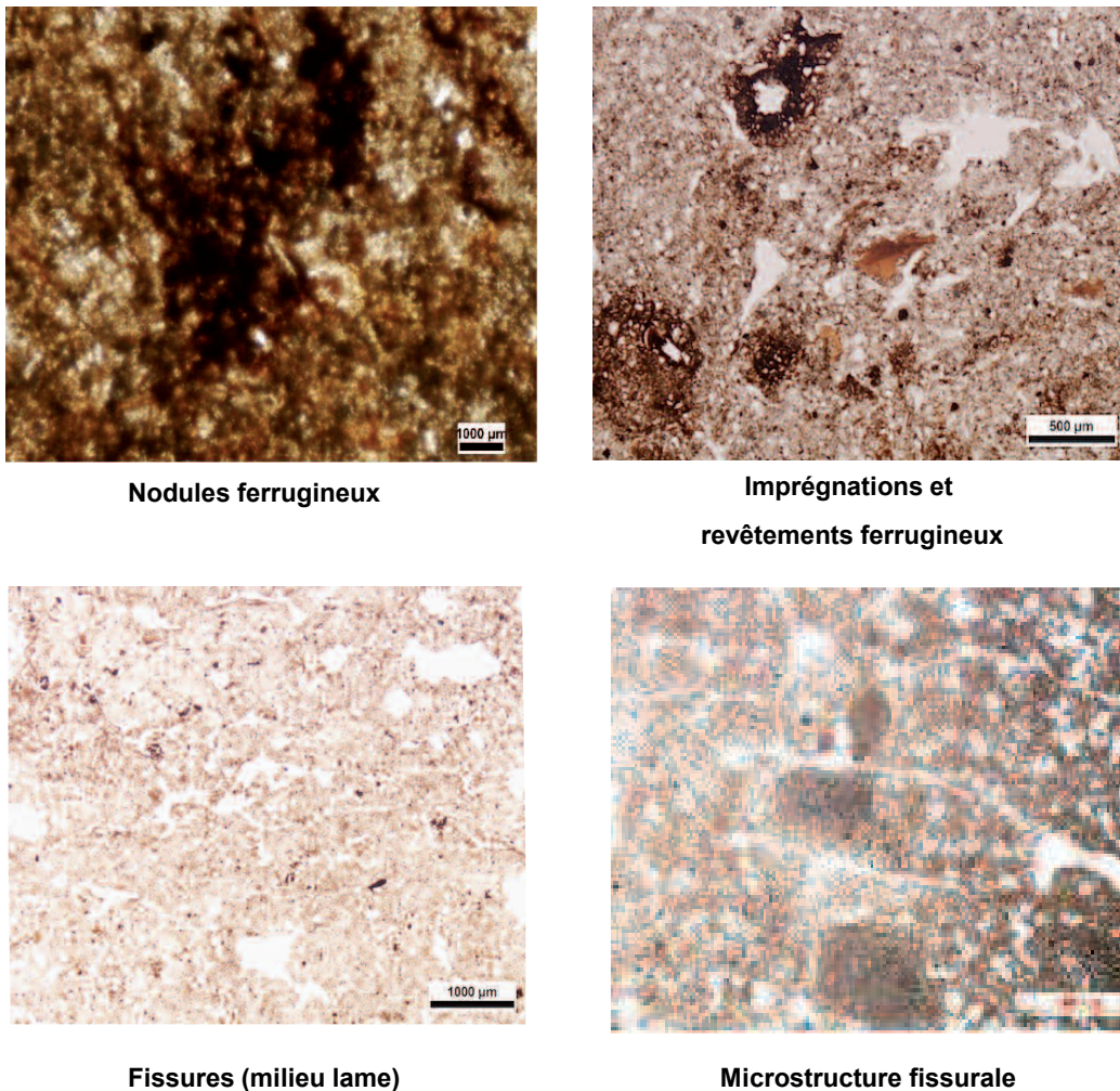
FIG. 8. — Clichés des traits ferrugineux et des fissures observées dans les lames minces. © M.-C. Charbonnier, C. Cammas, Inrap.
