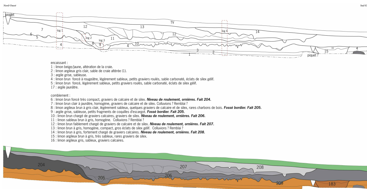
FIG. 7. — Relevé stratigraphique de la coupe 1 et localisation des échantillons micromorphologiques à Esclavolles-Lurey.
