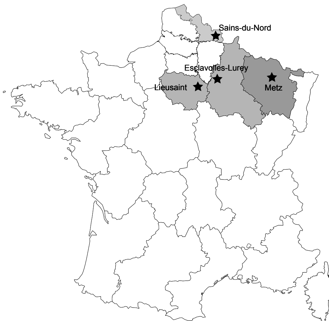
FIG. 1. — Localisation des sites de Sains-du-Nord, Metz, Lieusaint et Esclavolles-Lurey. © M.-C. Charbonnier, Inrap.
