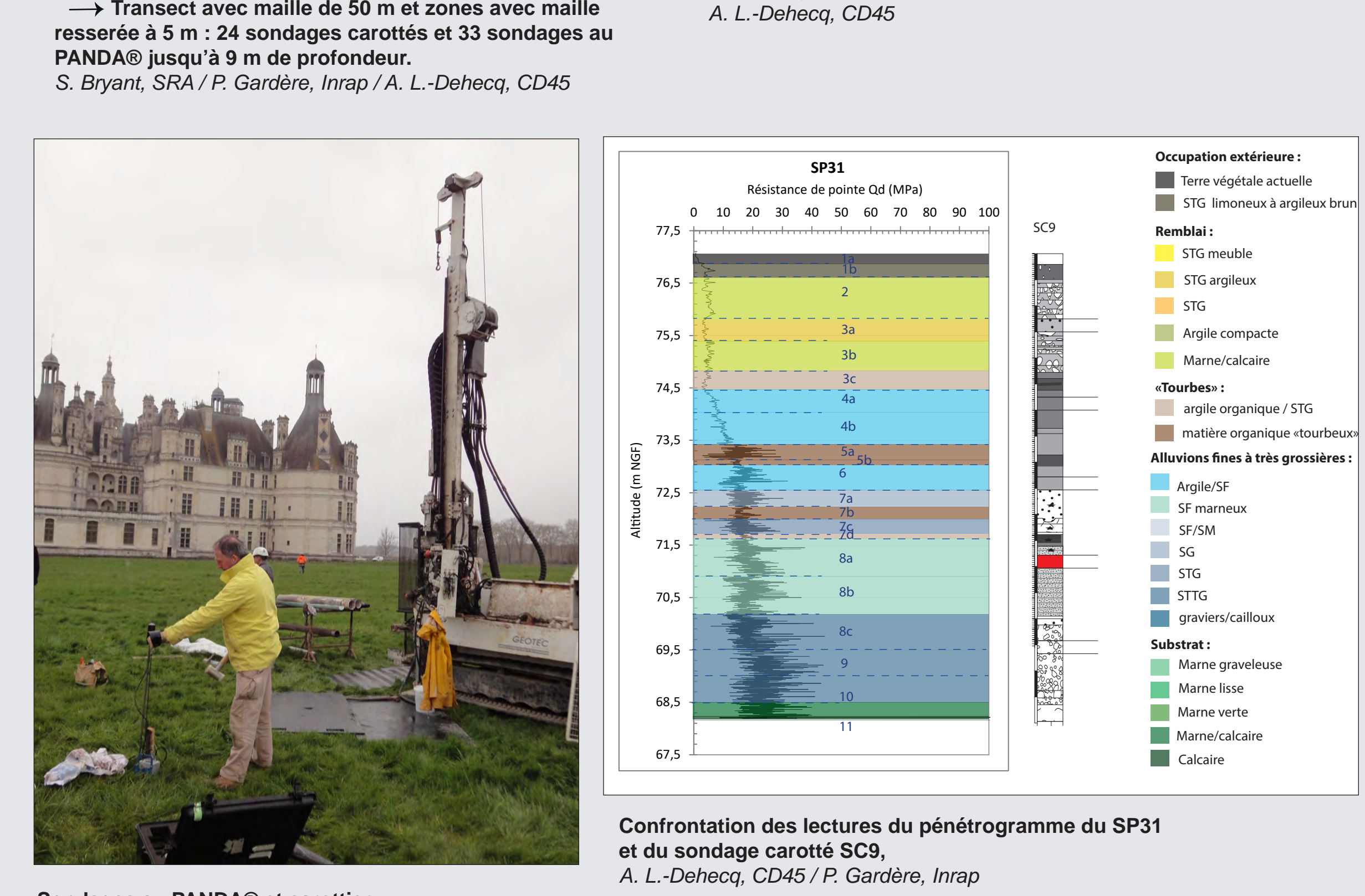
Confrontation des lectures du pénétrogramme du SP31 et du sondage carotté SC9. A. L.-Dehecq, CD45 / P. Gardère, Inrap
