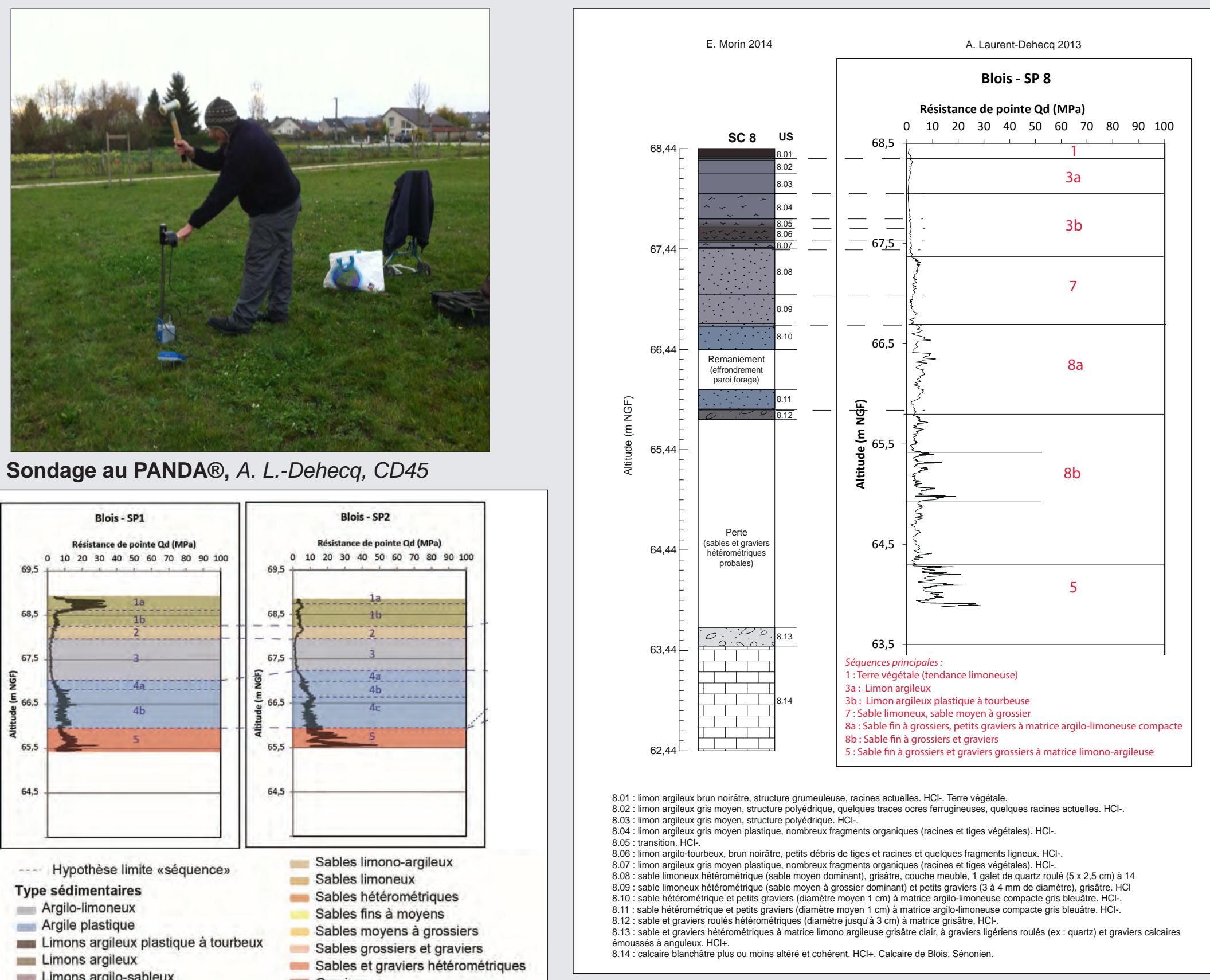
Extrait des pénétrogrammes (transect 1) et interprétations sédimentaires. A. L.-Dehecq, CD45 Confrontation des lectures du pénétrogramme du SP8 et du sondage carotté SC8. A. L.-Dehecq, CD45 / E. Morin, Inrap
