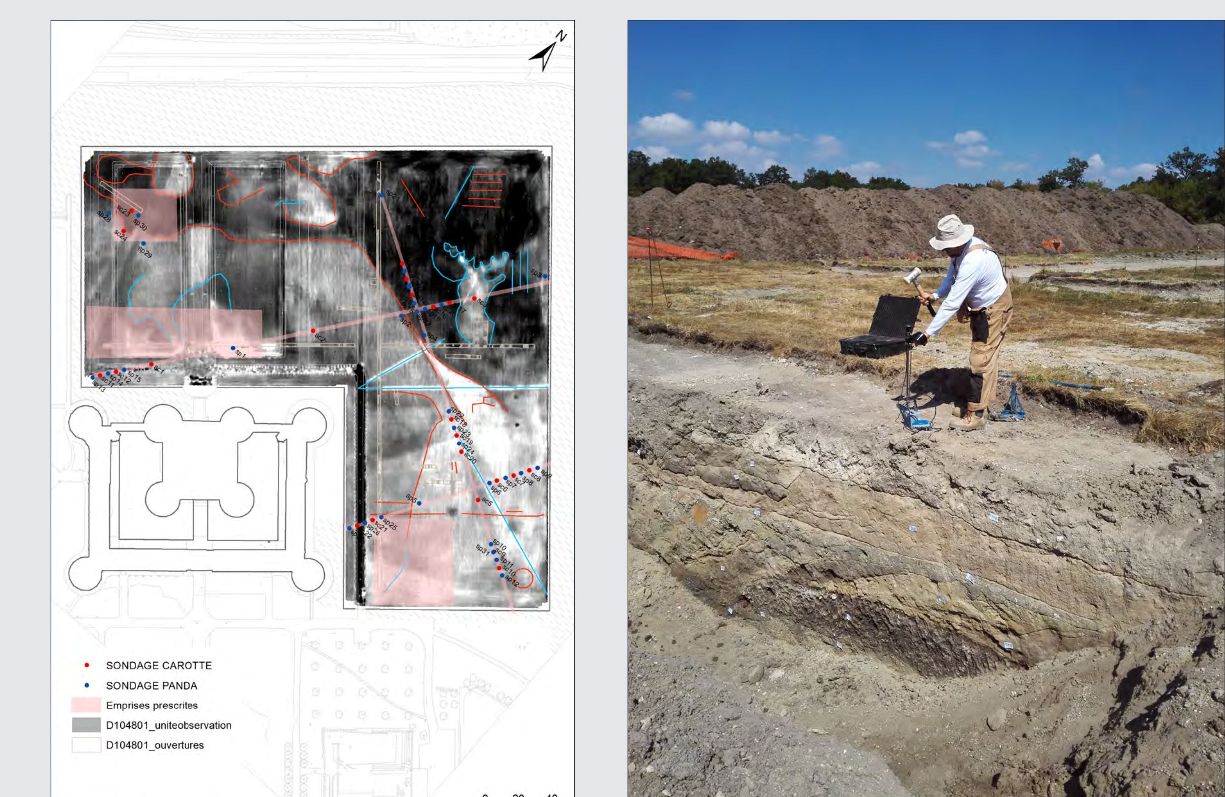
Prospection électrique ARP (prof. : 1,7 m / Géocarta, 2014) et transects réalisés en 2016. —> Transect avec maille de 50 m et zones avec maille reserrée à 5 m : 24 sondages carottés et 33 sondages au PANDA® jusqu'à 9 m de profondeur. S. Bryant, SRA / P. Gardère, Inrap / A. L.-Dehecq, CD45
